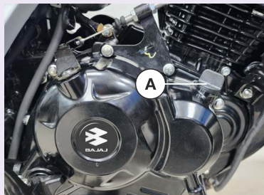
A : Oil Filler Cap
